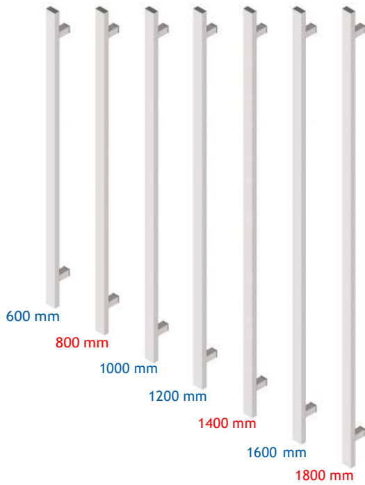
Q10 - Edelstahl Stangengriff 20x40
