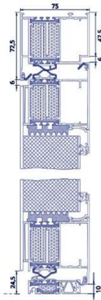
ProThermo 75 Plus Classic U_d=0,9 \text{ W/m}^2\text{K}
